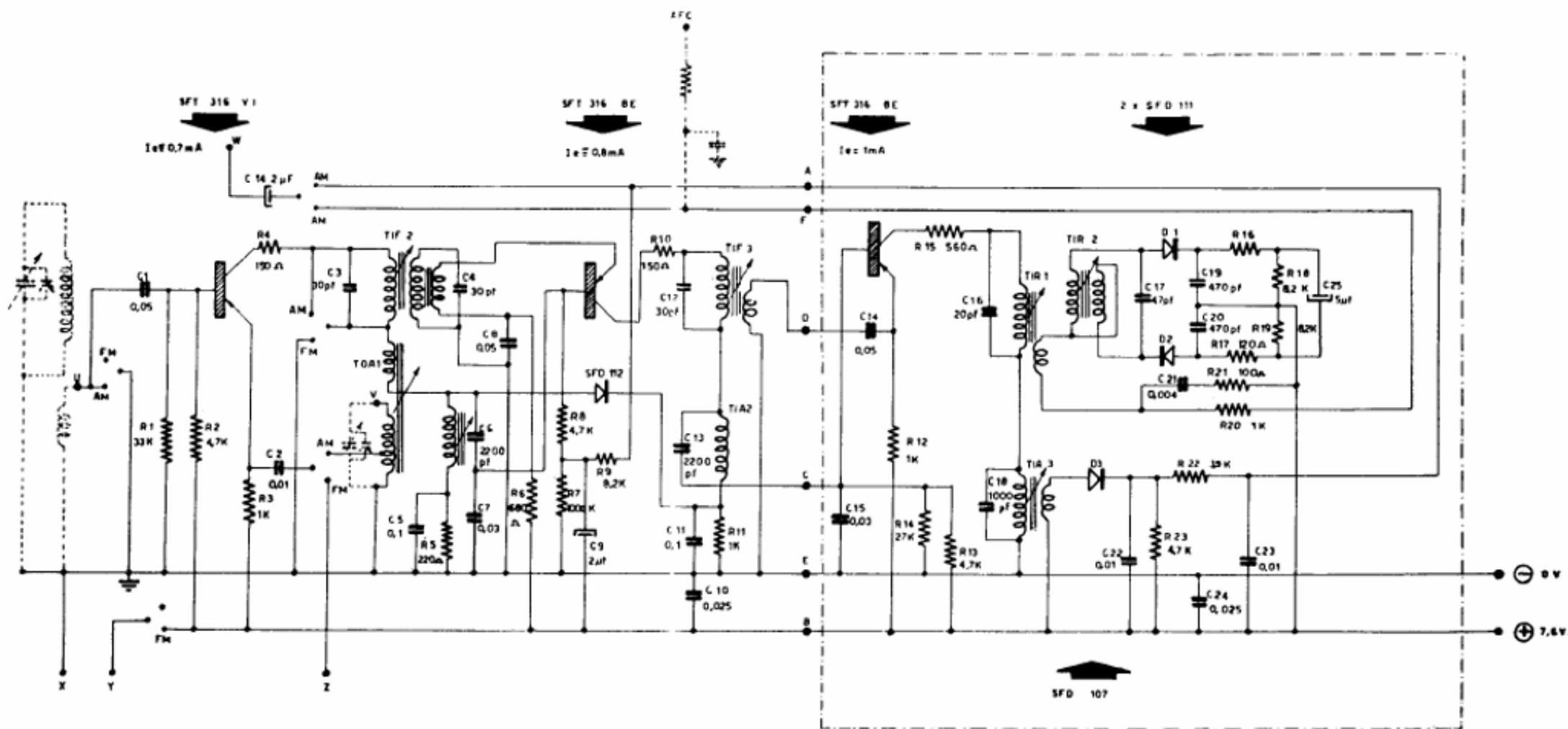
Schema elettrico del radiorecettore Atlantic mod T 398
